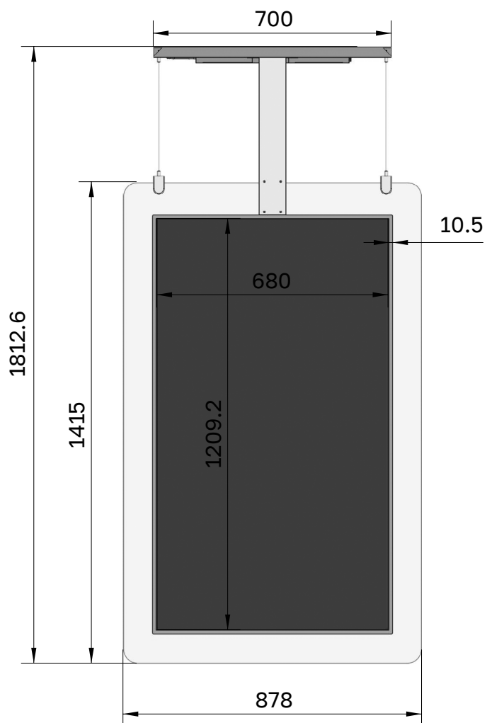
СХЕМА ДИСПЛЕЯ (ВИД СПЕРЕДИ)
